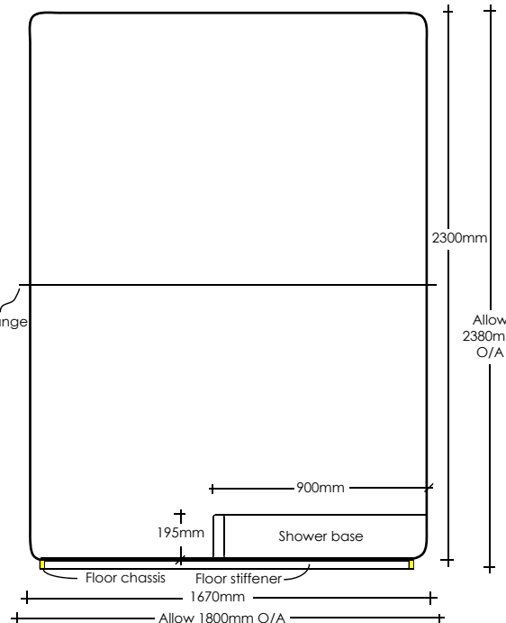
END ELEVATION
