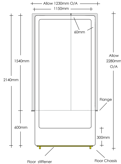
END ELEVATION
