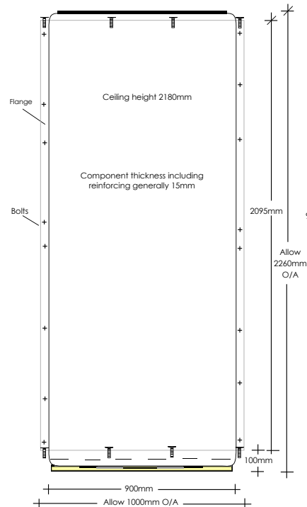
END ELEVATION
